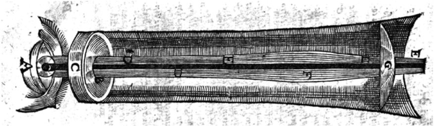
Afb. 23. De stralengang door een verrekijker volgens Girolamo Sirtori's Telescopium (1618)]
